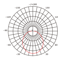
Rozkład natężenia światła
